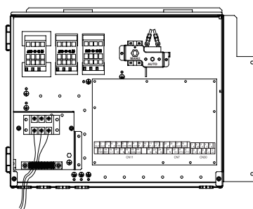
ZASILANIE JEDNOSTKI WEWNĘTRZNEJ Jednofazowa grzałka dodatkowa 6 kW
