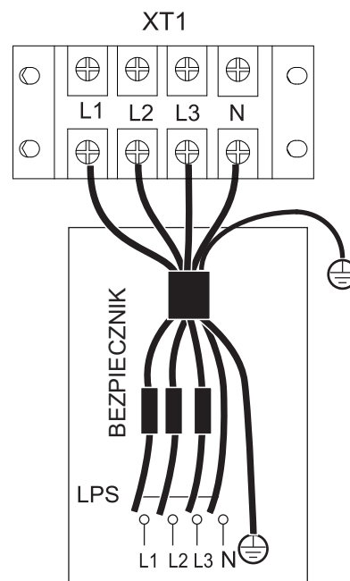
ZASILANIE JEDNOSTKI WEWNĘTRZNEJ Trójfazowa grzałka dodatkowa 9 kW
