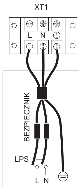
ZASILANIE JEDNOSTKI WEWNĘTRZNEJ Jednofazowa grzałka dodatkowa 6 kW
