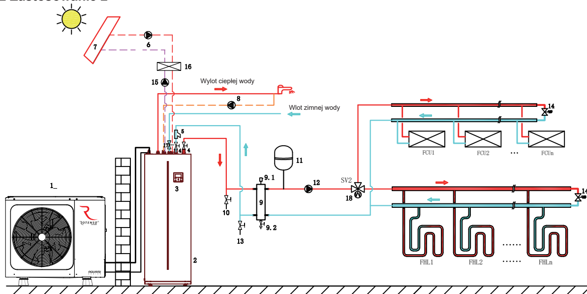
Jedna strefa dla pętli ogrzewania podłogowego i klimakonwektora
