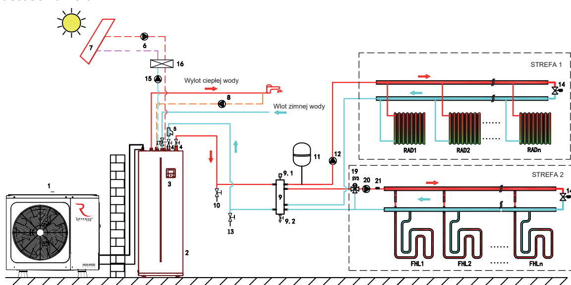
Podwójna strefa dla pętli ogrzewania podłogowego i grzejników
