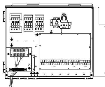
ZASILANIE JEDNOSTKI WEWNĘTRZNEJ Trójfazowa grzałka dodatkowa 9 kW
