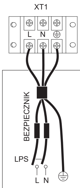
ZASILANIE JEDNOSTKI WEWNĘTRZNEJ Jednofazowa grzałka dodatkowa 3 kW
