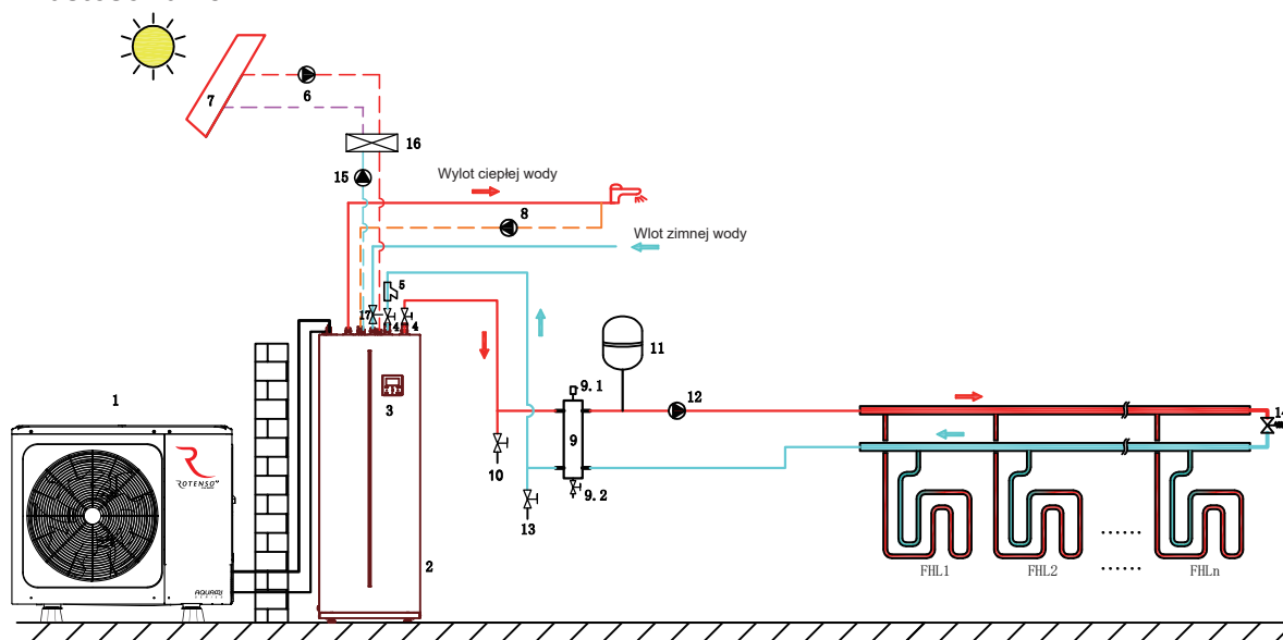
Jedna strefa dla pętli ogrzewania podłogowego
