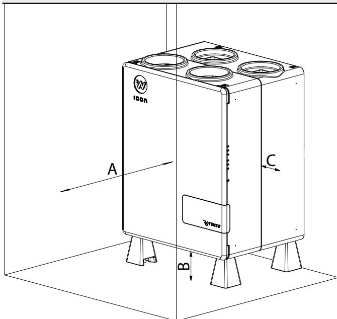
Opcja montażu - pionowa na stopach montażowych
