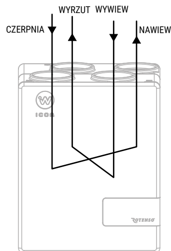
Schemat zasady działania wymiennika przeciwprądowego dla Standardowej (A) wersji wykonania.
